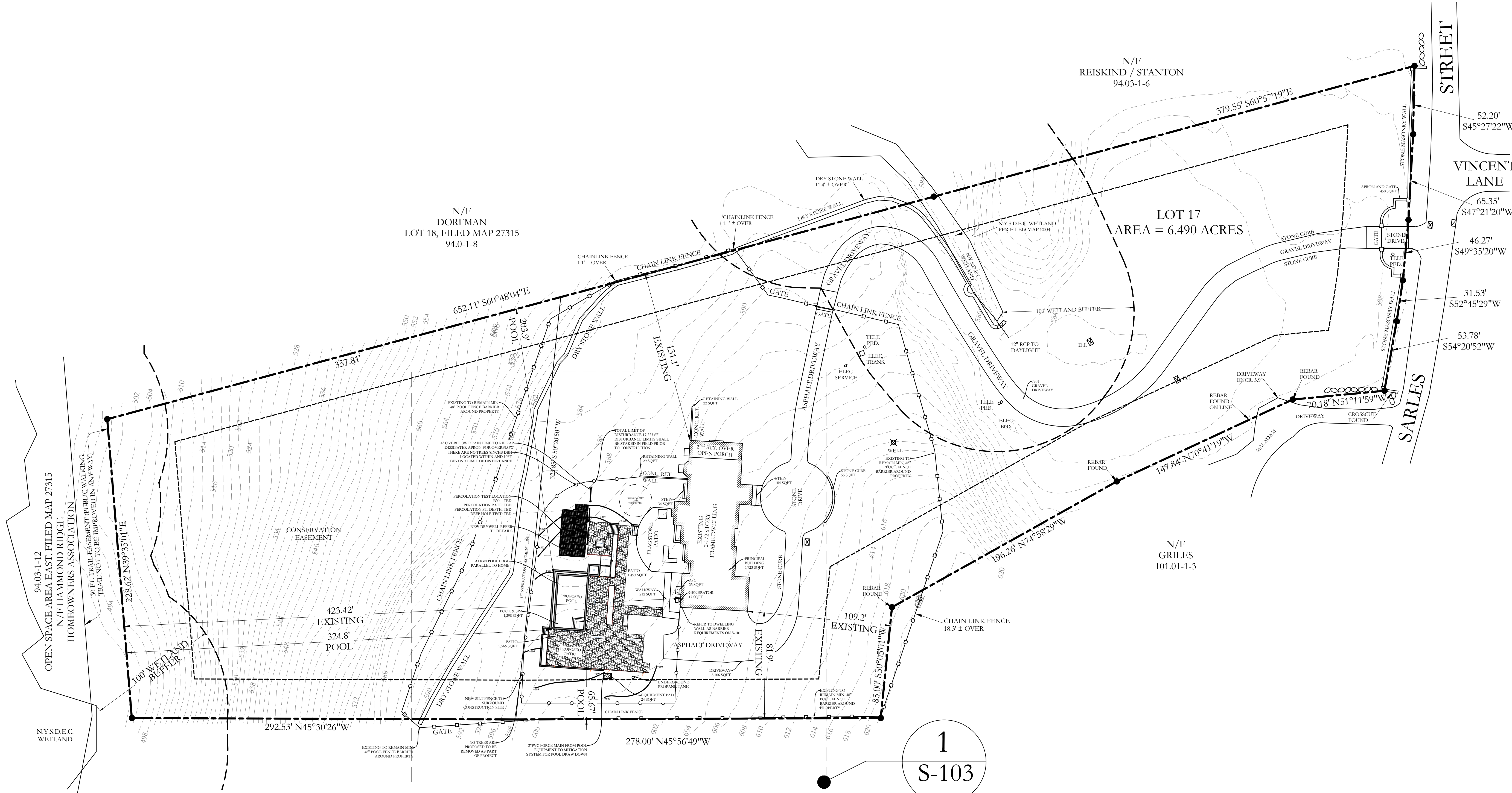
S-1 SITE PLAN SCALE: 1"=40'-0"
